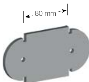
PT04 Staffa di collegamento tra pannello e muretto
