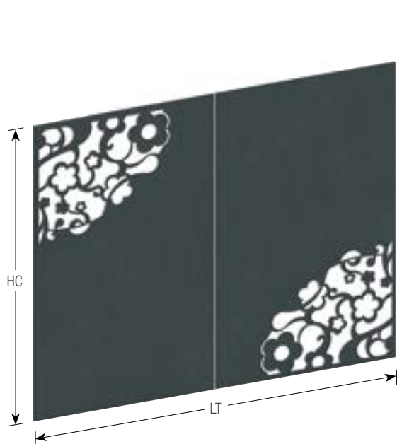
AUTO-2B | BATTENTE 2 ANTE AUTO-1S | SCORREVOLE Cancello
