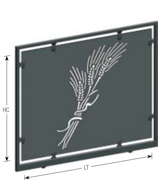
INT-2B | BATTENTE 2 ANTE INT-1S | SCORREVOLE Cancello
