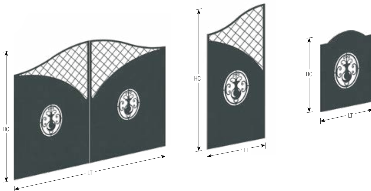
AUTO-2B | BATTENTE 2 ANTE AUTO-1S | SCORREVOLE Cancello
